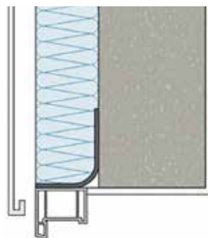
Figure 7 : Exemple de pose de menuiserie en applique extérieure
