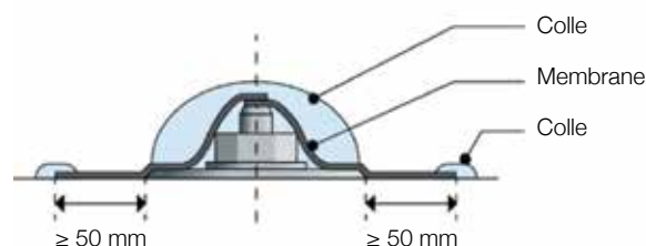
Figure 18 : Pontage au droit de pattes de fixation
