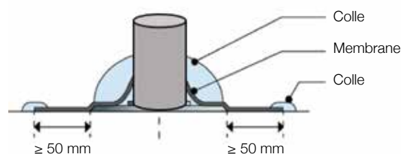
Figure 19 : Traversées diverses
